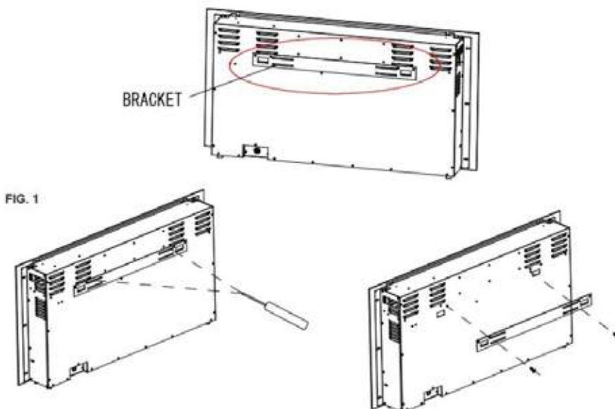
Illustration du support mural pour les modèles AV-WM42-50-60-65-72ROY
